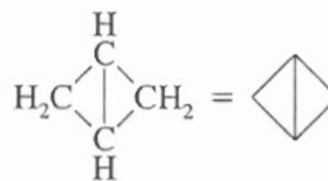
Bicyclo[1.1.0]butane
